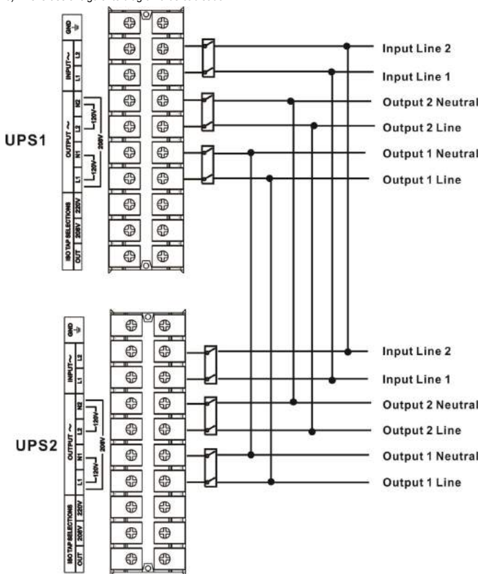
Diagrama de cableado del sistema en paralelo
